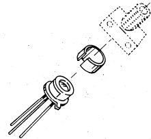
CASE 210A-01 METAL
